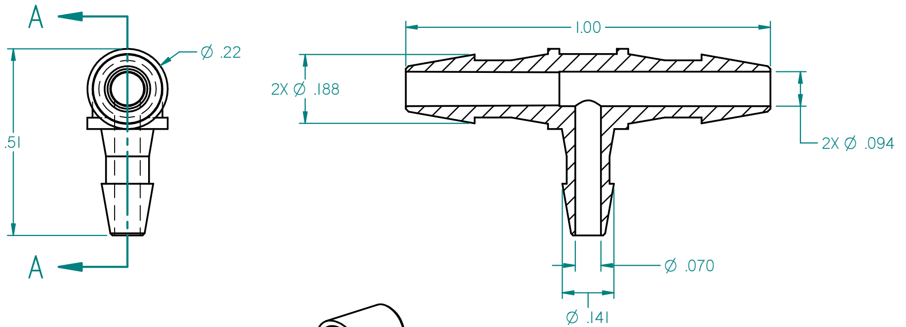
SECTION A-A
