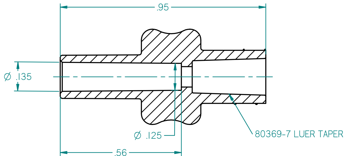
SECTION A-A
